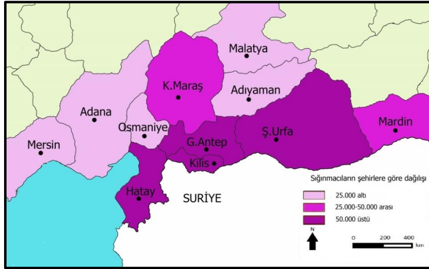
Harita 1: Suriyeli sığınmacıların illere göre yoğunluğu (BMMYK, 2014).
