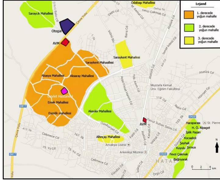
Harita 3: Sığınmacıların Hatay(Antakya)'da mahallelere göre dağılışı.
